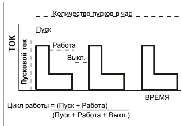
Рис. 9 Цикл работы, без шунтирования
