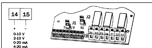
Рис. 37 Подключение аналогового сигнала
