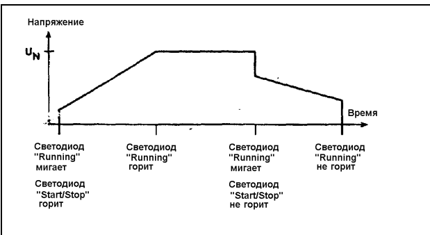
Рис. 14 Состояние светодиодов в различных режимах.
