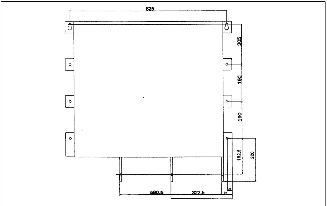
Рис. 23 Размеры отверстий для шин MSF-1000 ... MSF-1400
