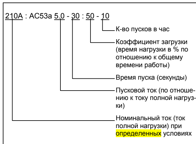
Рис. 8 Описание типоразмера по норме АС53а
