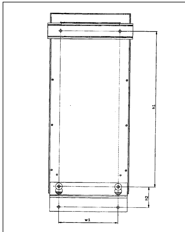
Рис. 17 Монтажные отверстия для MSF-017 ... MSF-250 (вид сзади).
