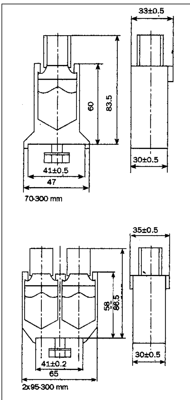
Рис. 64 Присоединительные клеммы
