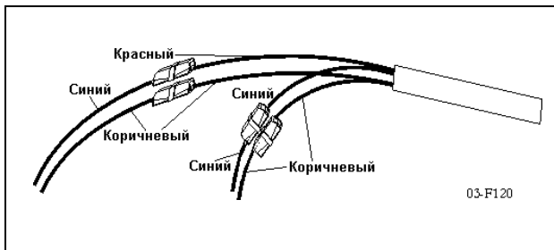
Рис. 63 Набор кабелей
