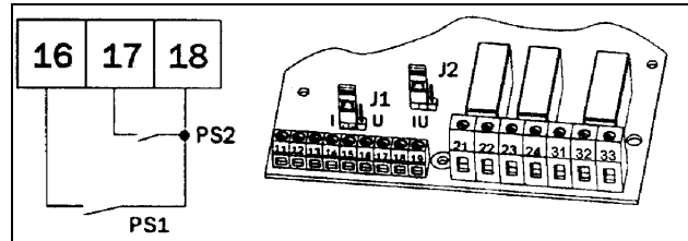
Рис. 56 Подключение сигналов управления
