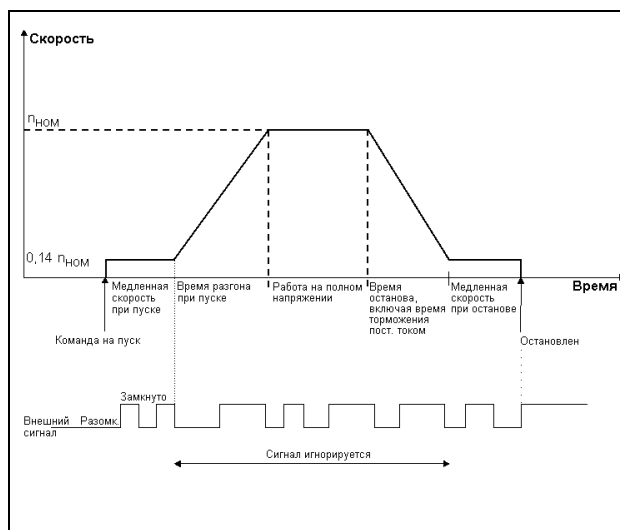
Рис. 48 Управление медленной скоростью при помощи внешнего сигнала.
