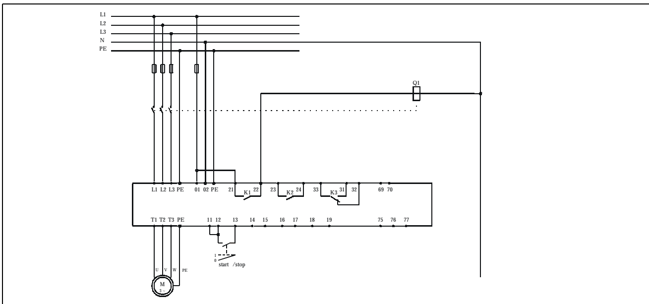
Рис. 6. Стандартное подключение
