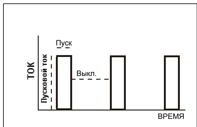
Рис. 11 Цикл работы, с шунтированием
