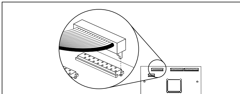
Fig. 11 Flatkabelpolarisering.
