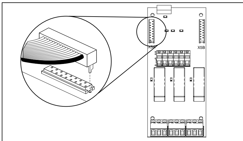
Fig. 18 Anslut flatkabeln till X5A-anslutningen på tillvalskortet.
