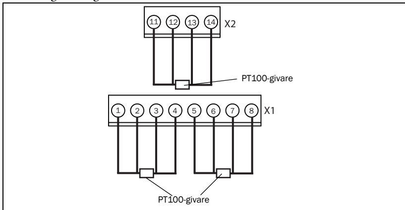
Fig. 8 Anslutning av PT100-givare för 4-ledars temperaturmätning.
