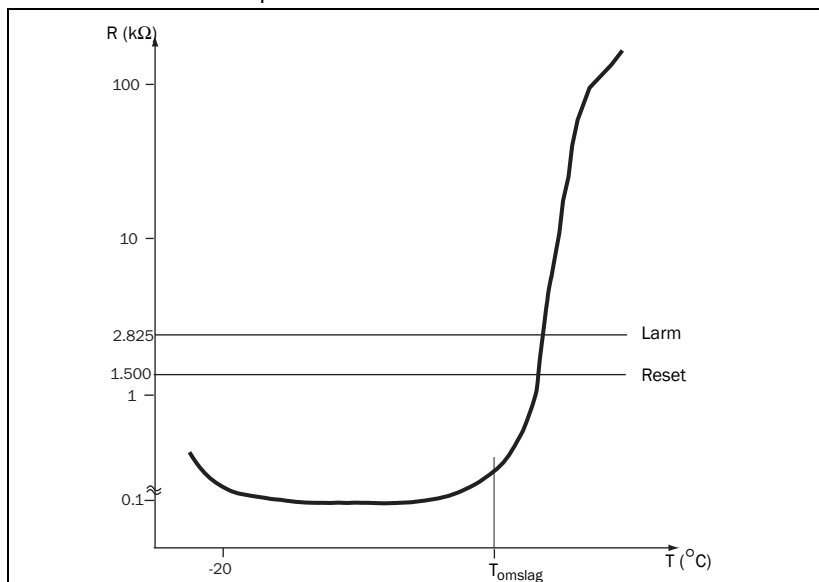
Fig. 4 Typisk PTC-kurva
