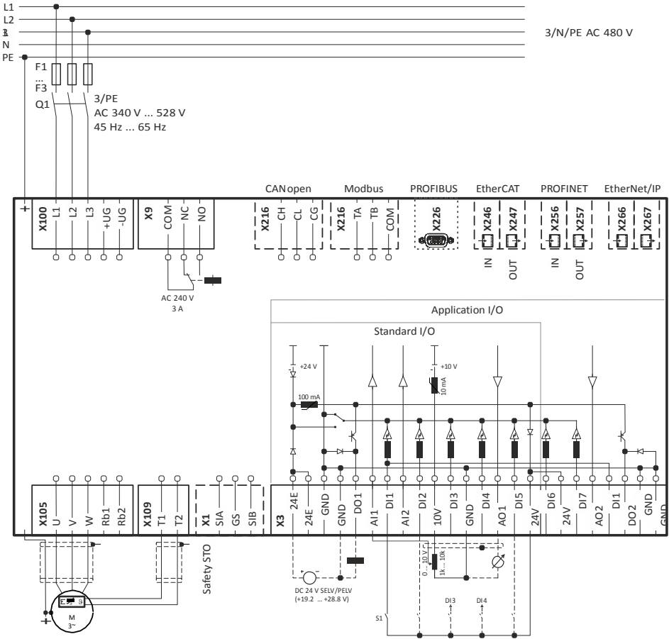
Fig. 2: Wiring example
